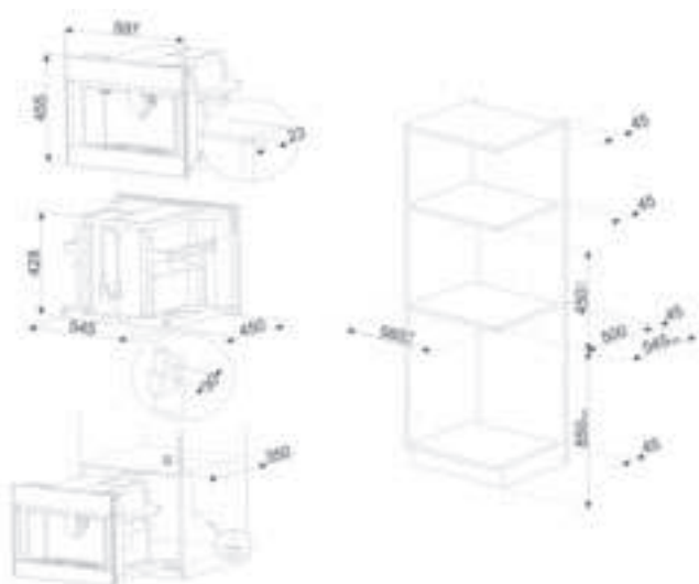
MACCHINE DA CAFFÈ
