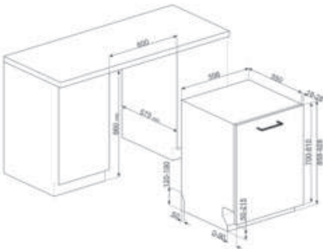
LAVASTOVIGLIE ALTEZZA 86 CM ANTA LUNGA: STL324AQLH, STL332CH, STL252CH
