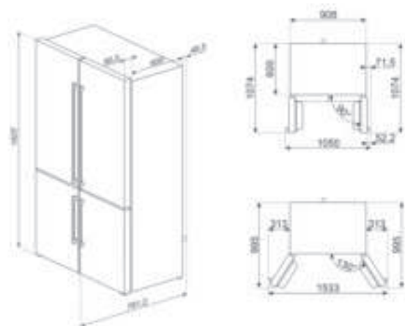
FQ60XDAIE, FQ60XDE, FQ60NDE, FQ60BDE, FQ60XE
