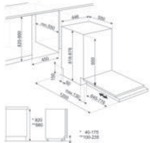
LAVASTOVIGLIE LARGHEZZA 45 CM: ST4523DIN, ST4512EIN
