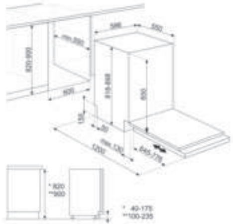
LAVASTOVIGLIE LARGHEZZA 60 CM: STL361DQ
